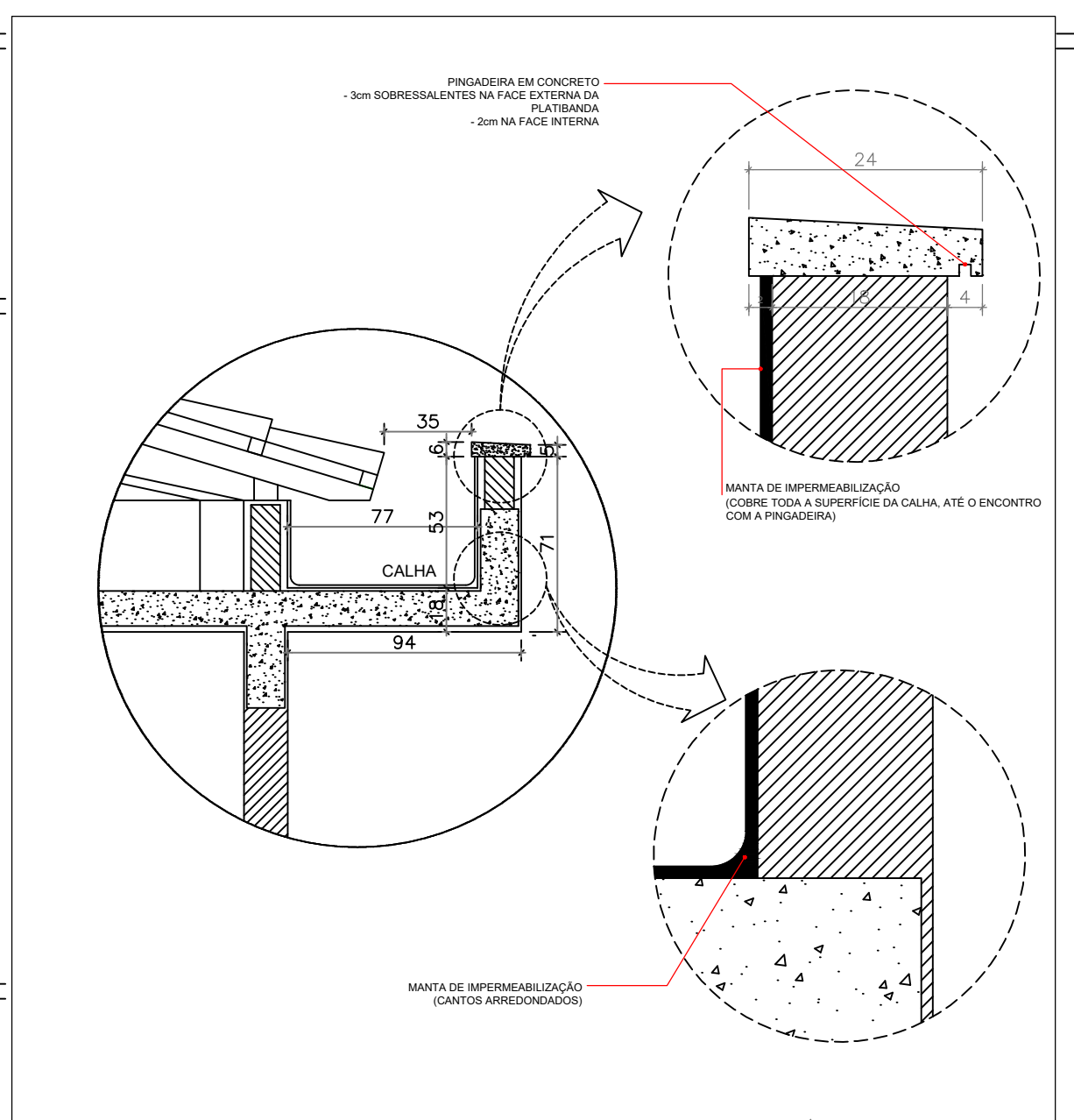
DETALHE: CALHA E PLATIBANDA
